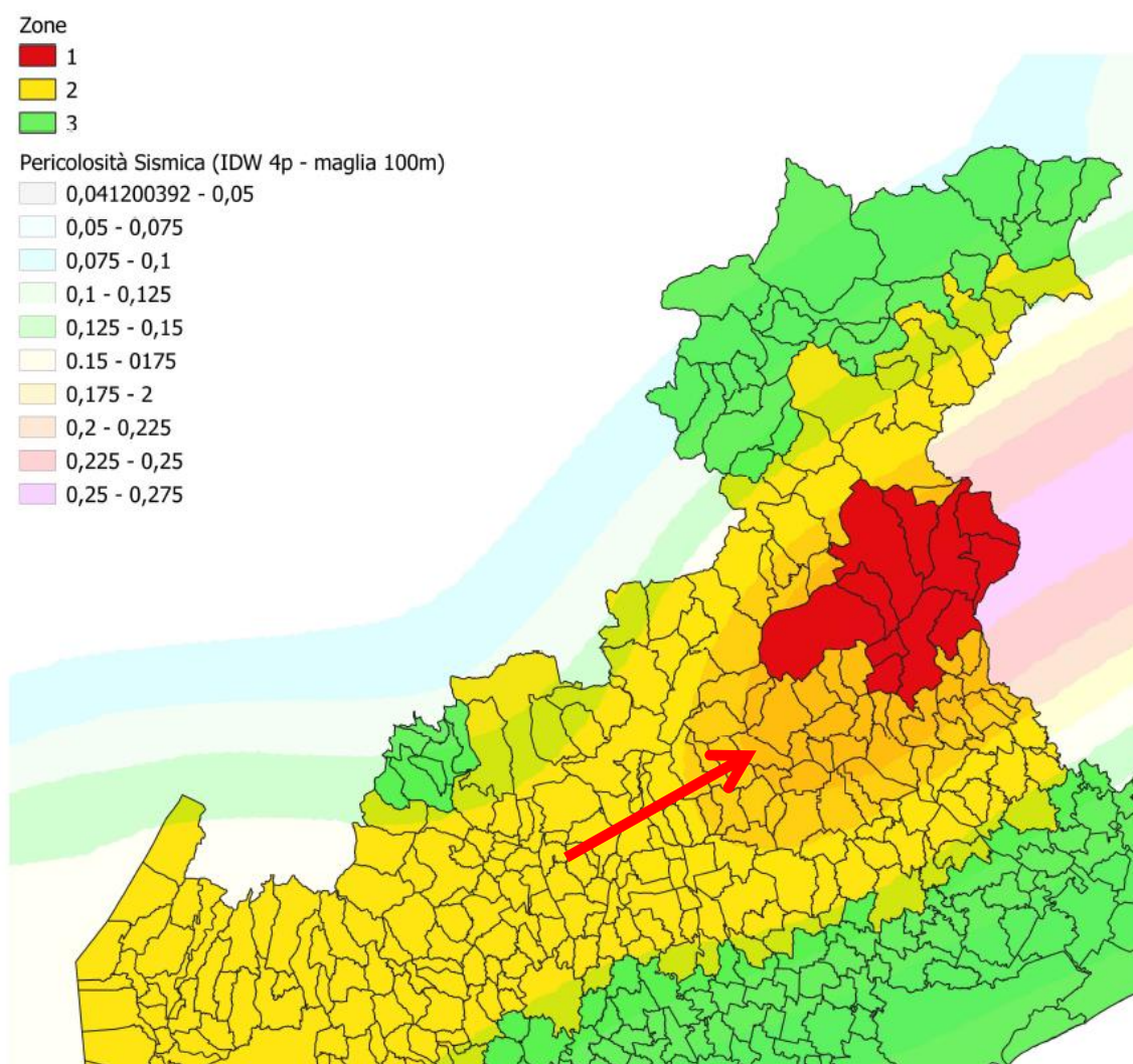
Fig. 2.4 – estratto della Zonizzazione Sismica di cui alla DRGV n. 244 del 09/03/2021 Classificazione sismica del Veneto Mappa di pericolosità sismica
